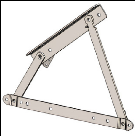
STAN Midi Sandık Mekanizma
